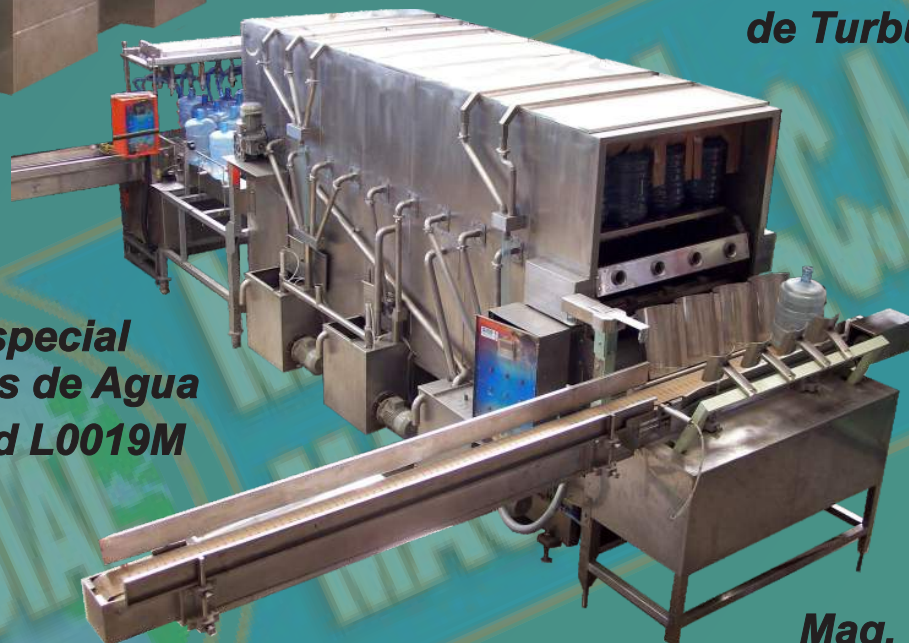
Lavadora Industrial de Turbulencia
